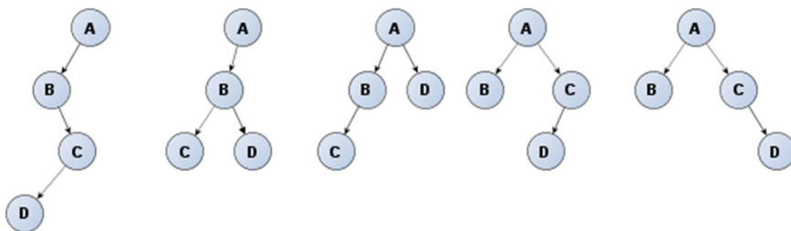
Erinevaid kahendpuid, mille tippude töötlemise järjekord eesjärjestuses on ABCD
