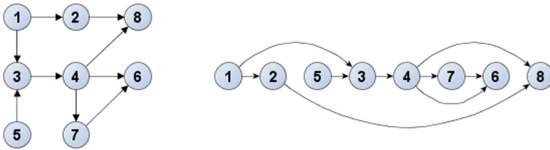
Suunatud graaf ja selle topoloogiliselt sorteeritud esitus
