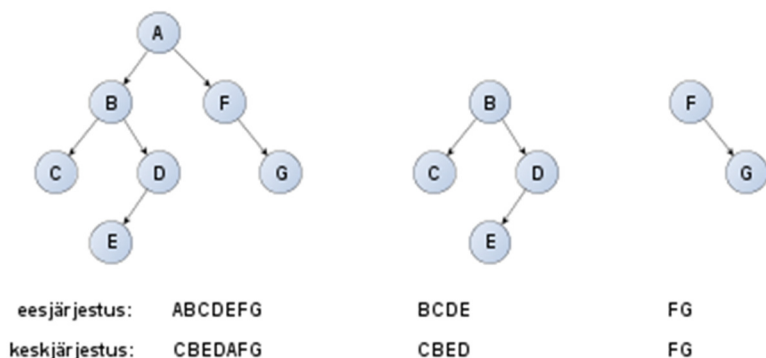
Vasakul on puu juurega A, keskel selle vasakpoolne alampuu ja paremal parempoolne alampuu
