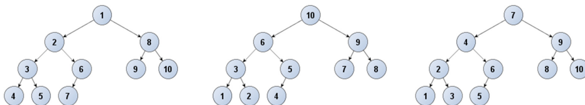
Puu läbimine ees-, lõpp- ja keskjärjestuses. Numbrid tippudes tähistavad läbimise järjekorda.
